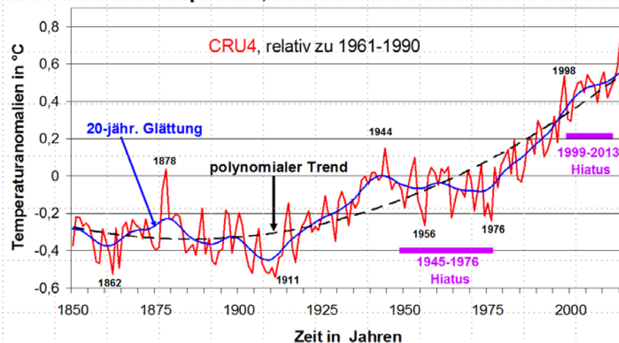
Globaltemperatur, Jahresanomalien 1850 - 2016
